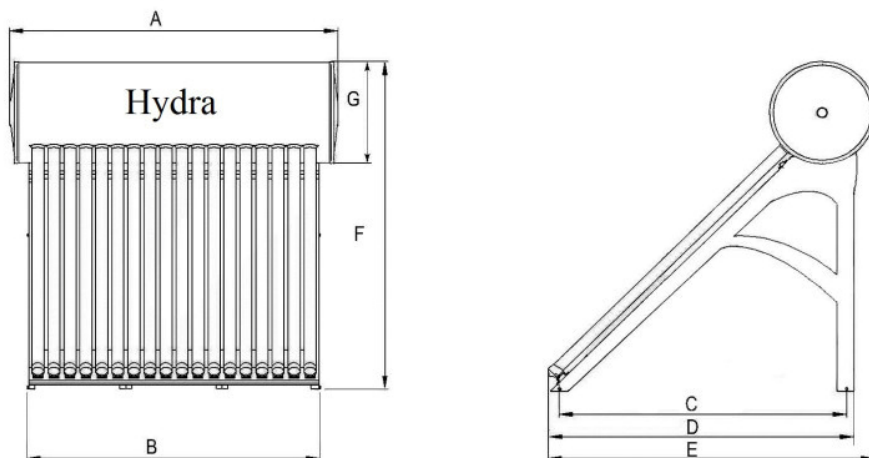
Rozmiary oraz wagi podgrzewaczy z serii PROECO HYDRA
