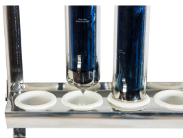
profil przedni dolny – (element 8 ) oraz plastikowe uchwyty do rur próżniowych
